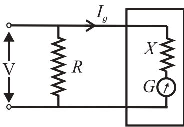
Fig. 9.14 : Voltmeter.
