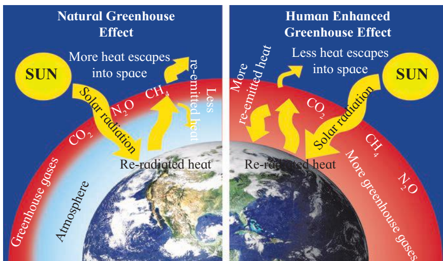
Fig. 15.10 : Greenhouse effect
